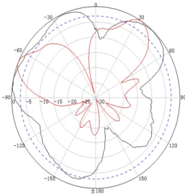
1710MHz
