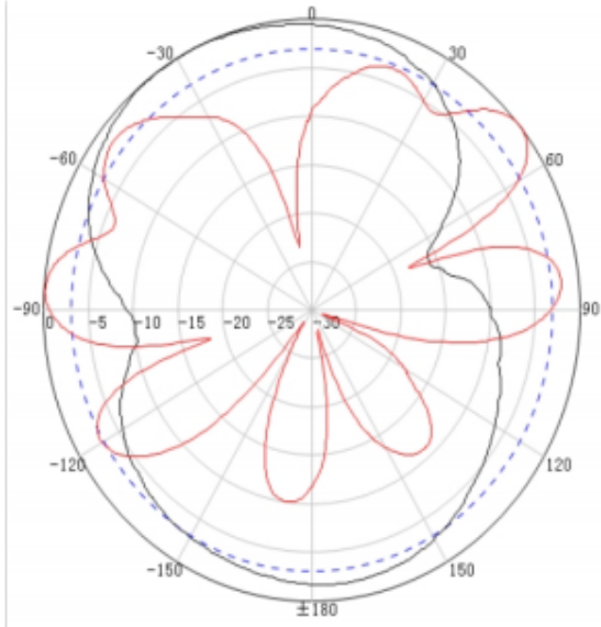
700MHz
