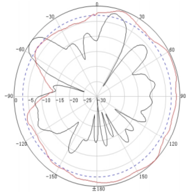
2700MHz
