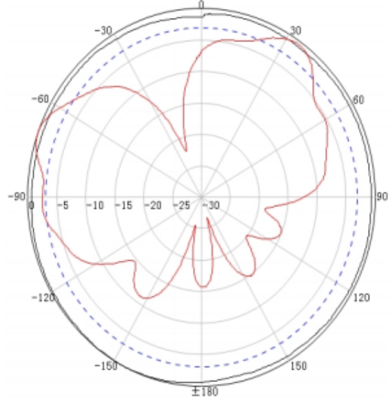
960MHz
